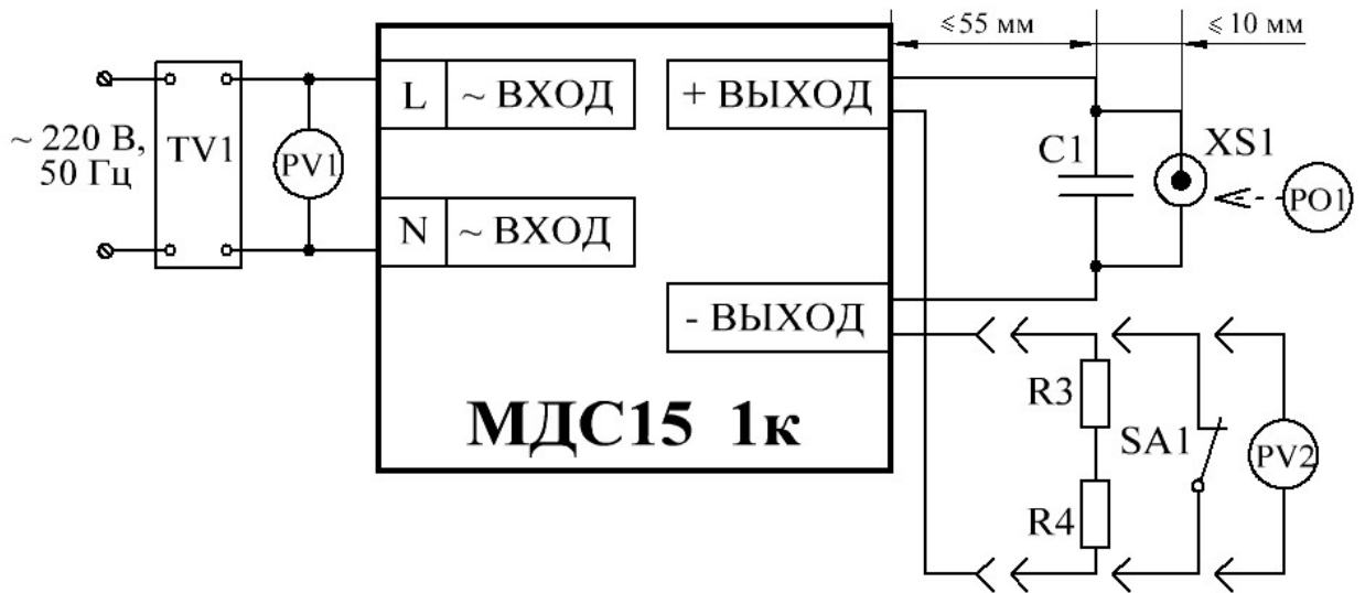
Рисунок Г.1 – Схема проверки амплитуды пульсации выходного напряжения модулей
