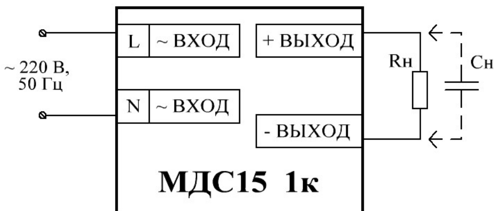
Рисунок Д.1 – Типовая схема включения модулей
