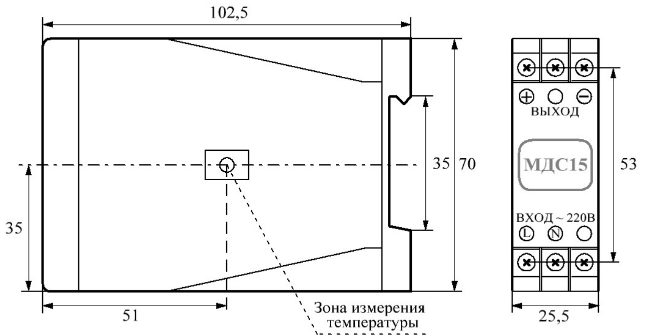
Рисунок Ж.1 – Точка измерения температуры корпуса модулей
