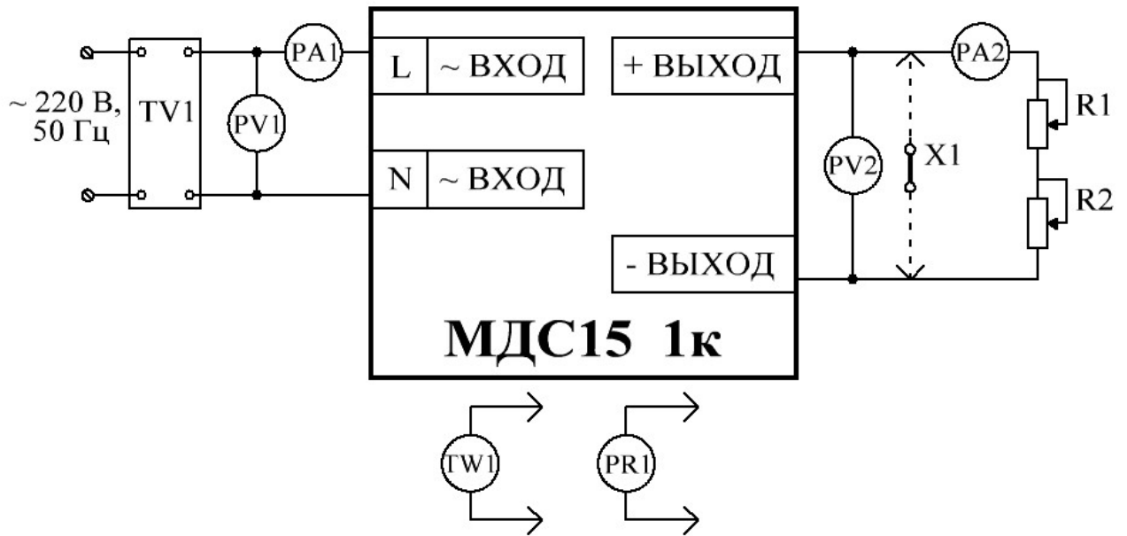
Рисунок В.1 – Схема проверки электрических параметров модулей
